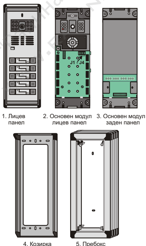
Фиг. 28 Механичен монтаж на отделните елементи RN-255C5:
