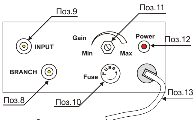
Заден панел
