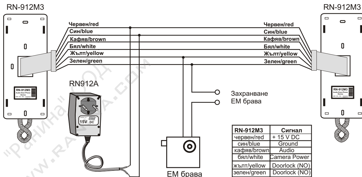
Фиг. 27 Свѡрзване на два аудиодомофона RN-912M3.
