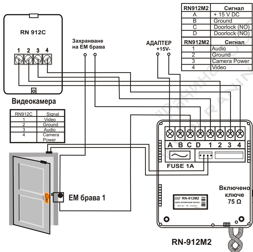
Фиг. 28 Свѡрзване на видеокамера RN-912C с видеомонитор RN-912M2
